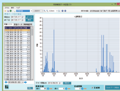
1時間雨量 1週間表示
