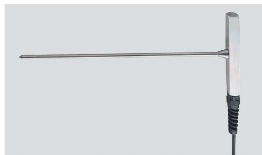
●SK-S109K アスファルト用センサ 0~300°C φ5×L250mm (材質:SUS304) コード1.1m付 No. 8080-40 ¥15,700 (税抜き) (センサ精度 クラス2)
