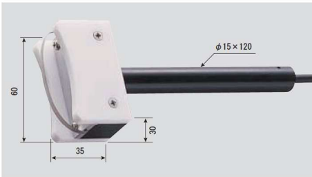
●SK-S401K 曲面表面用 (パイプ等) 0~250°C 先端部30×35×60mm コード1.1m付 No. 8080-70 ¥17,200 (税抜き) (センサ精度 クラス2)
