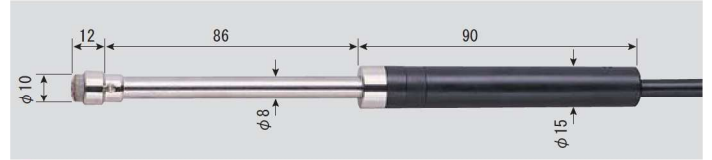
●SK-S306K 静止表面用 (低温) -30~250°C 先端部φ10×L12mm コード1.1m付 No. 8080-60 ¥13,700 (税抜き) (センサ精度 クラス2)
