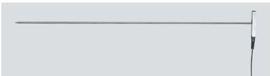
●SK-S108K 堆肥用センサ 0~300°C φ8×L900mm (材質:SUS304) コード1.1m付 No. 8080-38 ¥18,200 (税抜き) (センサ精度 クラス2)
