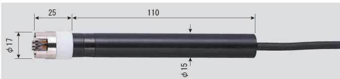
●SK-S307K 静止表面用 (一般計測、低温) -30~400°C 先端部φ17×L25mm コード1.1m付 No. 8080-62 ¥13,700 (税抜き) (センサ精度 クラス2)
