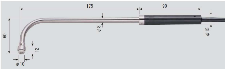
●SK-S303K 静止表面用L型 (中・高温用) 0~800°C 先端部φ10×L12mm コード1.1m付 No. 8080-54 ¥13,700 (税抜き) (センサ精度 クラス2)
