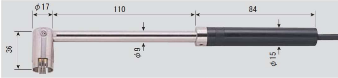
●SK-S305K 静止表面用 (90° 角度可変、中温) -30~500°C 先端部φ17×L36mm コード1.1m付 No. 8080-58 ¥20,200 (税抜き) (センサ精度 クラス2) (写真は90°に曲げた状態)
