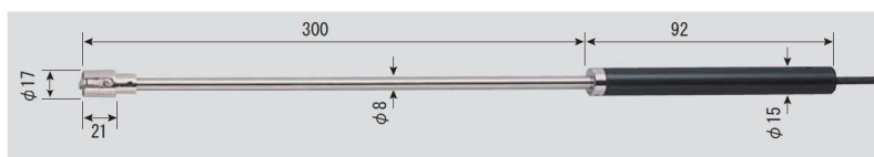
●SK-S302K 静止表面用 (ロングサイズ) 0~600°C 先端部φ17×L21mm コード1.1m付 No. 8080-52 ¥21,200 (税抜き) (センサ精度 クラス2)
