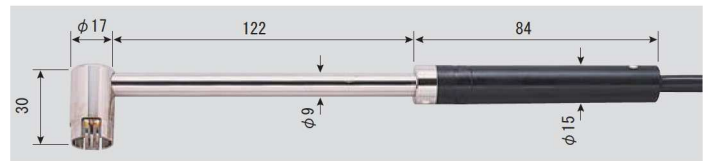
●SK-S308K 静止表面用 (L型センサ、中温) -30~600°C 先端部φ17×L30mm コード1.1m付 No. 8080-64 ¥15,700 (税抜き) (センサ精度 クラス2)
